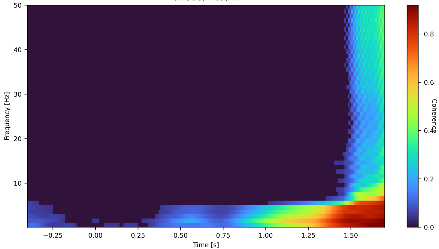
dPFC (F3) - PEC (P7)
